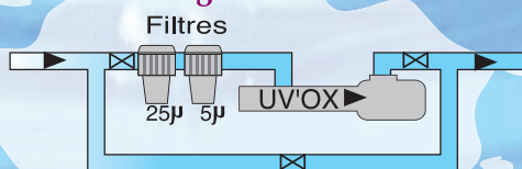
Montage horizontal
